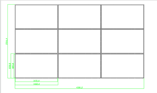
裸眼3D (3*3) 拼接屏尺寸示意图
